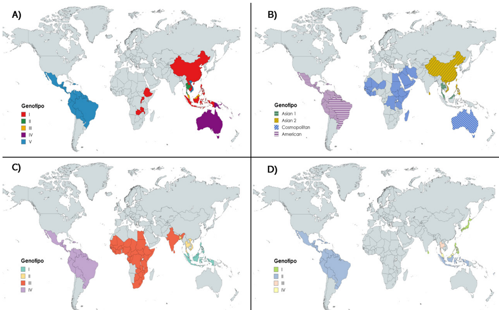
Figura 3. Distribución Geográfica de los Genotipos y serotipos de DENV. A) DENV-1 B) DENV-2 C) DENV-3 D) DENV-4 (Harapan et al. , 2020)
